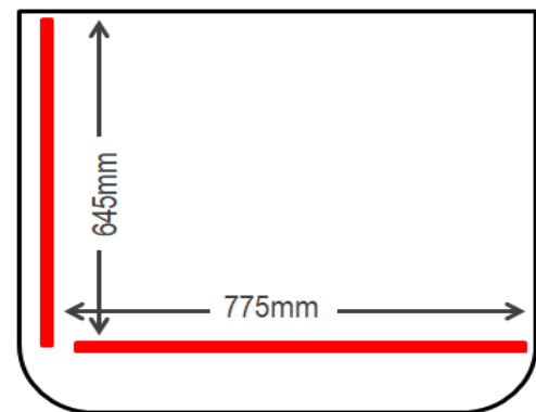
Detalle de barras de sellado en cámara de vacío.
